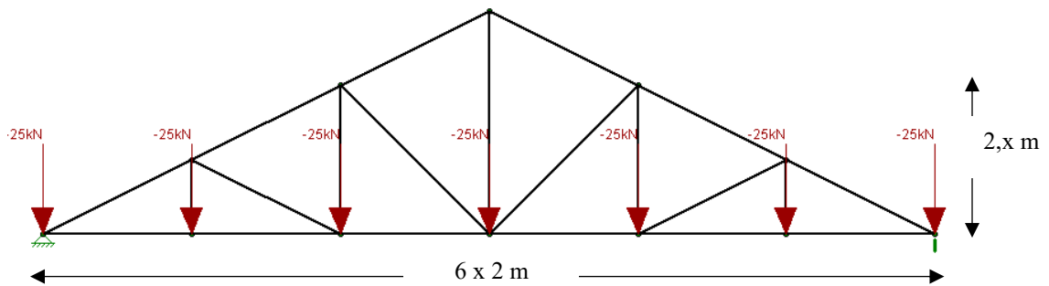
a. Rangka kuda-kuda
