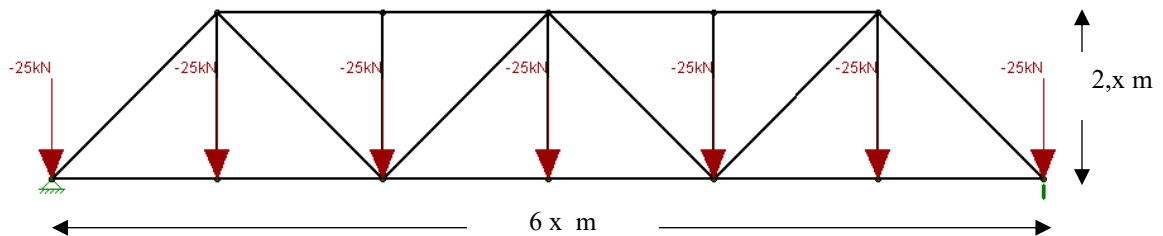
b. Rangka Jembatan
